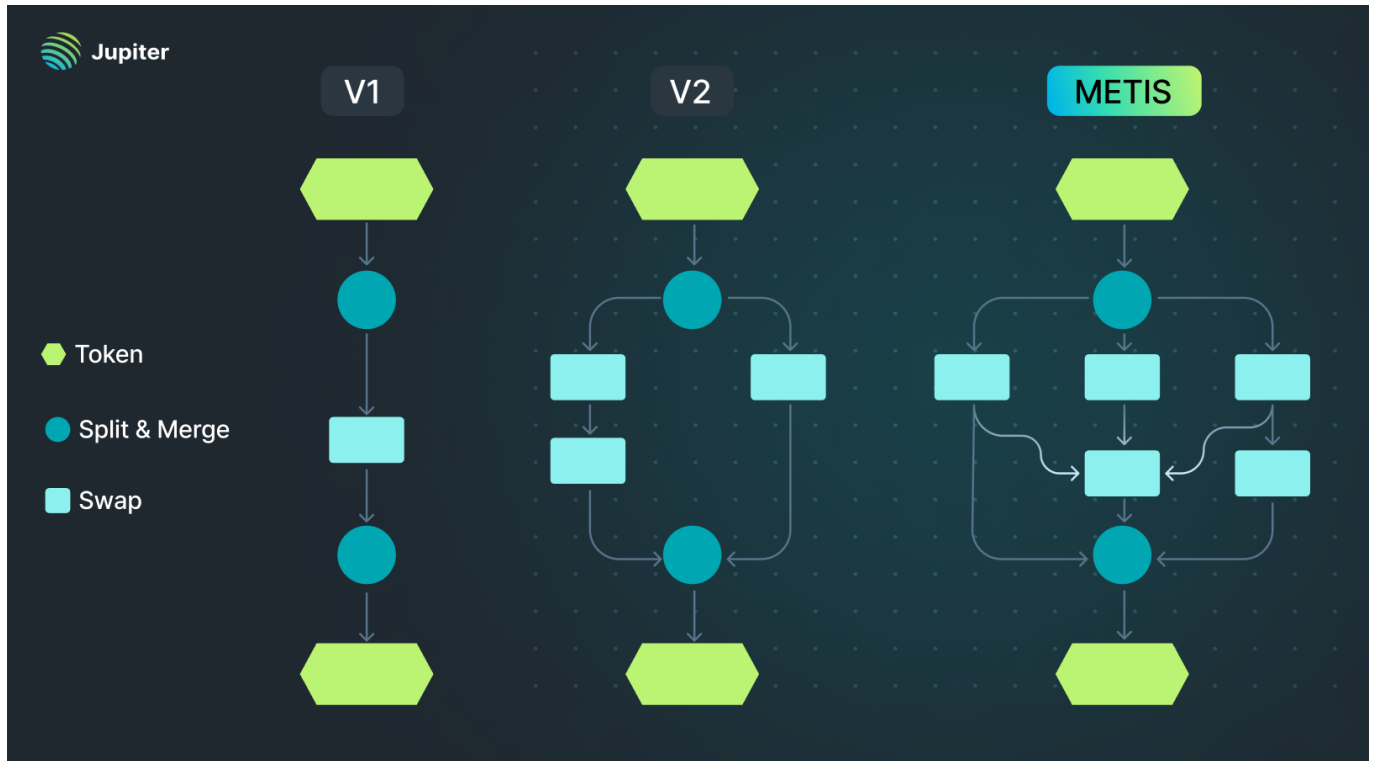
[메티스 라우팅 알고리즘]
